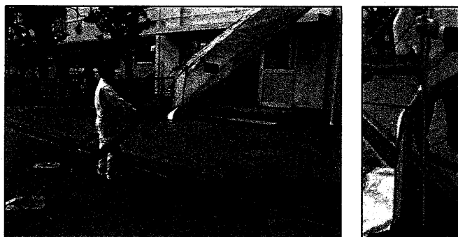
古い斜降式救助袋に関する検証実験の様子 ※7
